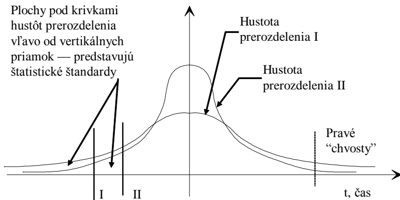
Obr. 4. Obsah plôch pod krivkami prerozdelenia I a II od -\infty až po zvislé priamky I a II je rovnaký, takže pri jednom a tom istom štatistickom štandarde dostávame na časovej osi dva rozdielne kontrolné body . Vo vzťahu k tej istej krivke hustoty prerozdelenia každá zo zvislých priamok I a II zodpovedá vlastnej hodnote štatistického štandardu.
