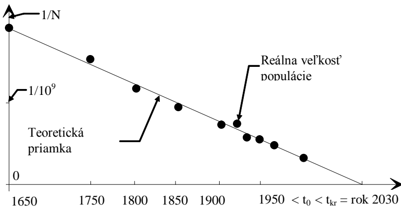
Obr. 2. Porovnanie známych reálnych hodnôt priebežnej súhrnnej počtosti ľudstva ( N ) v dostatočne známych a dobre naštudovaných epochách ( t ) s príslušným prirodzeným — teoreticky očakávaným — hyperbolickým zákonom nárastu populácie: N(t) = N(0)/(1 - t/t_{kr}) , t.j. dN/dt \sim N^2 .
